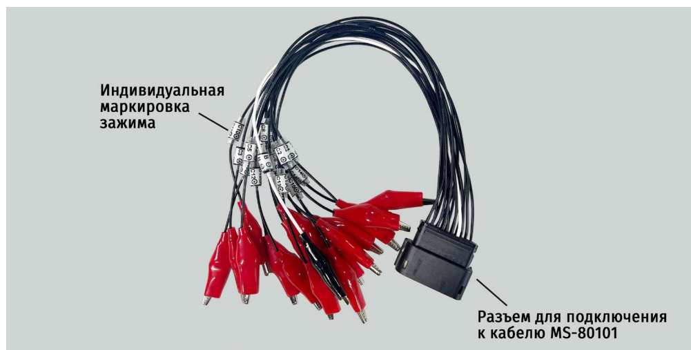
Рисунок 3. Общий вид универсального кабеля-переходника
