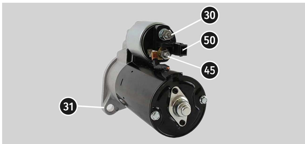
Rysunek 31. Położenie клем na rozruszniku
