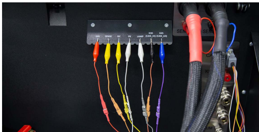
Рисунок 7. Зажимы универсального диагностического кабеля, зафиксированные на держателе.
