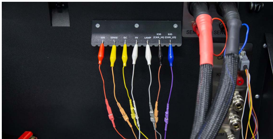
Rysunek 7. Zaciski kabla diagnostycznego zamocowane na uchwycie
