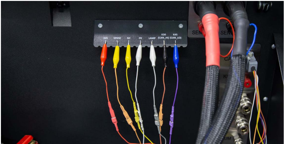
Figura 7. Abrazaderas de cable de diagnóstico universal fijadas en el soporte
