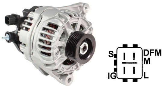
Abbildung 20. Generator Toyota 2706020230 und Bezeichnung der Anschlüsse im Stecker
