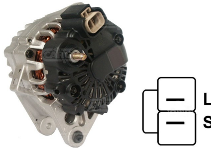
Abbildung 19. Generator Bosch 0986049191 und Bezeichnung der Anschlüsse im Stecker
