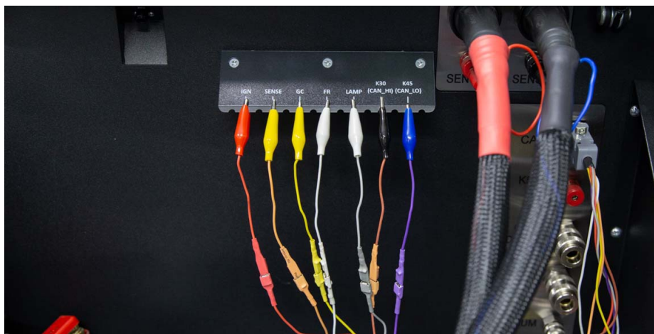
Abbildung 7. Am Halter befestigte Krokodilklemmen des universellen Diagnosekabels.
