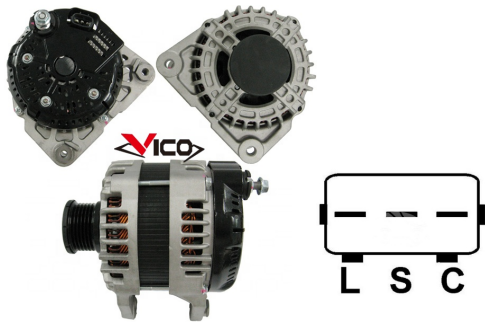
Abbildung 21. Generator Nissan 23100EN000 und Bezeichnung der Anschlüsse im Stecker
