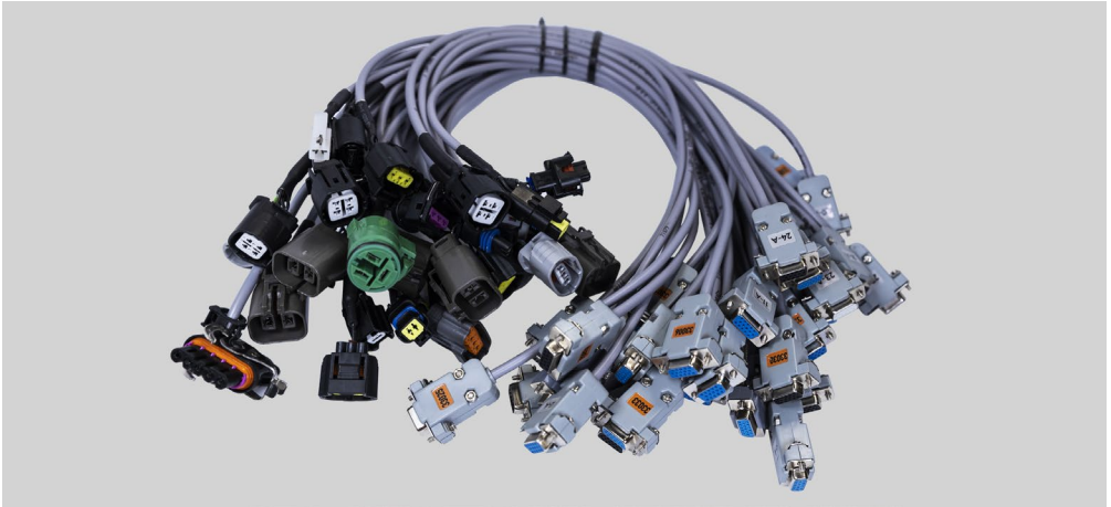
Abbildung 9. Spezialkabel zur Diagnose von Generatoren 12/24 V
