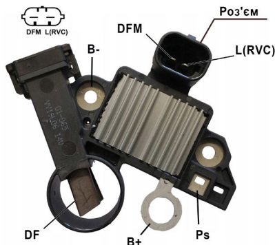
Рисунок 18. Регулятор ARE1054
