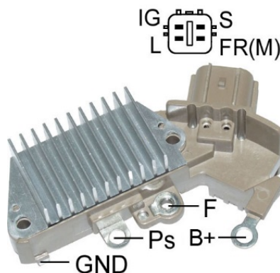
Рисунок 19. Регулятор ARE6076
