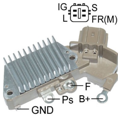
Рисунок 20. Регулятор ARE6076
