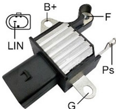
Рисунок 22. Регулятор ARE6149P
