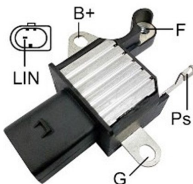
Figura 22. Regulador ARE6149P
