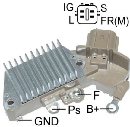
Figura 20. Regulador ARE6076
