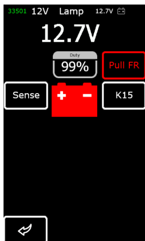
Figura 14. Pantalla de diagnóstico del alternador/regulador del tipo Lamp (12 / 24V)
