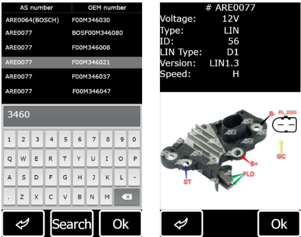
Figura 17. Búsqueda de regulador en la base de datos y resultados de la búsqueda Conecte el cable de diagnóstico al regulador según el diagrama.
