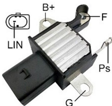
Figura 23. Regulador ARE6149P
