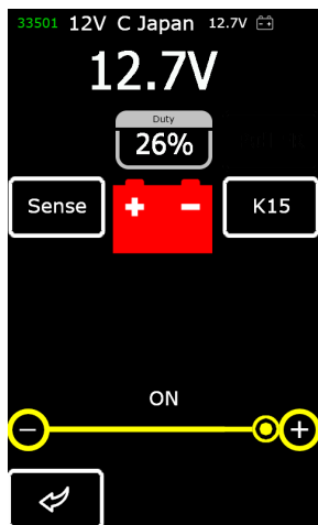
Figura 13. Pantalla de diagnóstico del alternador/regulador del tipo C JAPÓN
