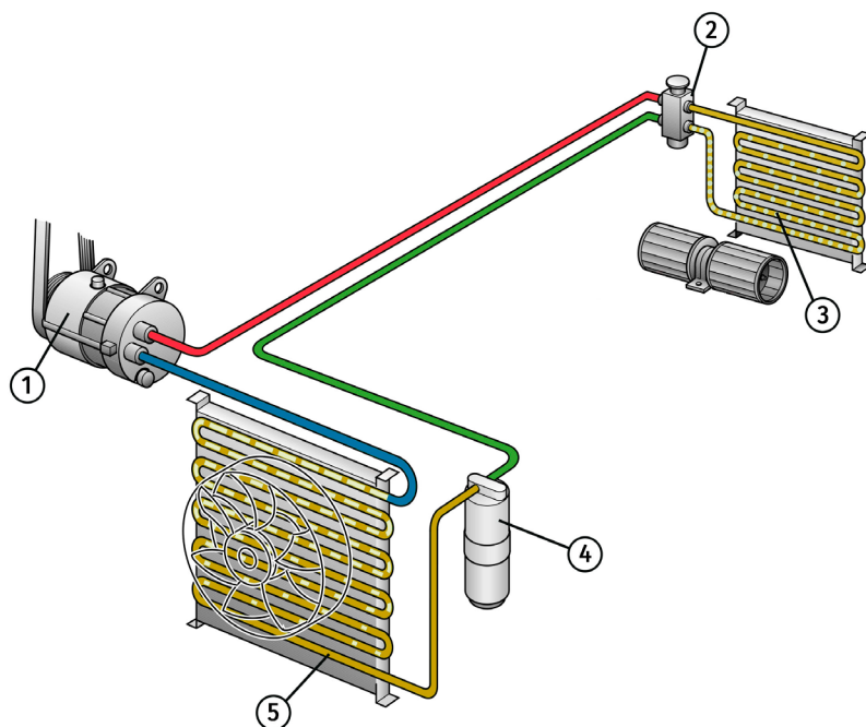
Figura 3. Esquema del sistema de aire acondicionado del vehículo:
