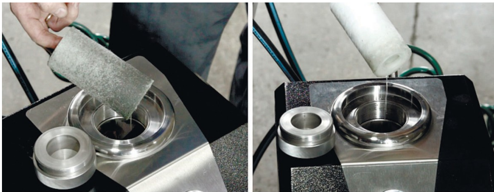
Figura 4. Elemento filtrante después del primer ciclo de lavado (a la izquierda) y al finalizar el lavado (a la derecha).
