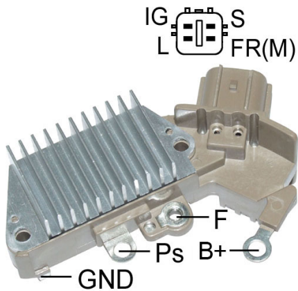
Figura 17. Regulador ARE6076
