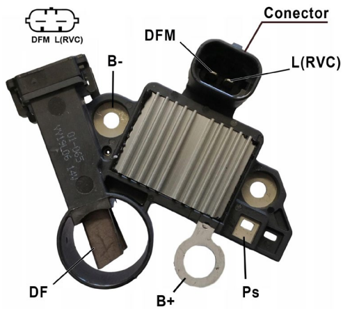
Figura 15. Regulador ARE1054
