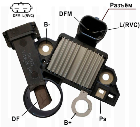
Рисунок 15. Регулятор ARE1054
