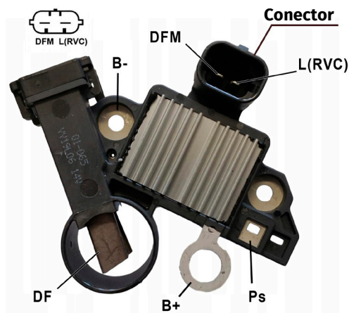
Figura 15. Regulador ARE1054
