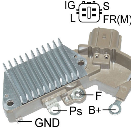
Figura 17. Regulador ARE6076
